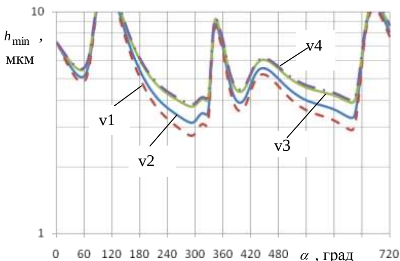
Рис. 15. Зависимость минимальной толщины смазочного слоя от угла поворота коленчатого вала
