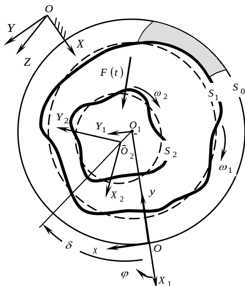
Рис. 1. Сечение подшипника
