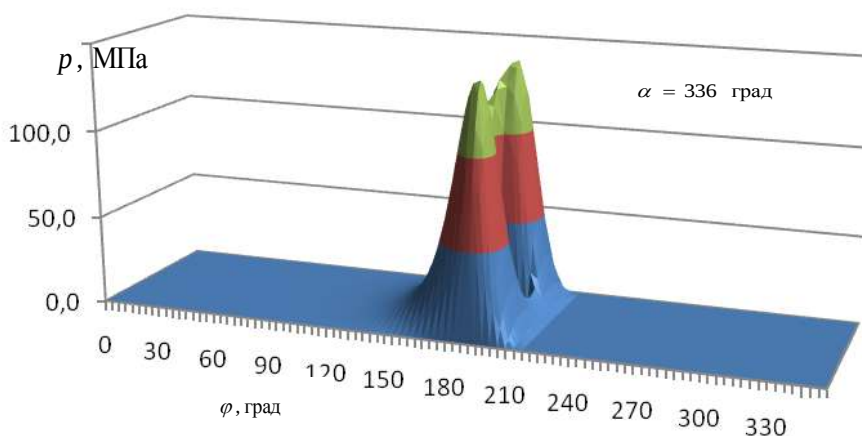
Рис. 13. Эпюры распределения гидродинамических давлений в смазочном слое
