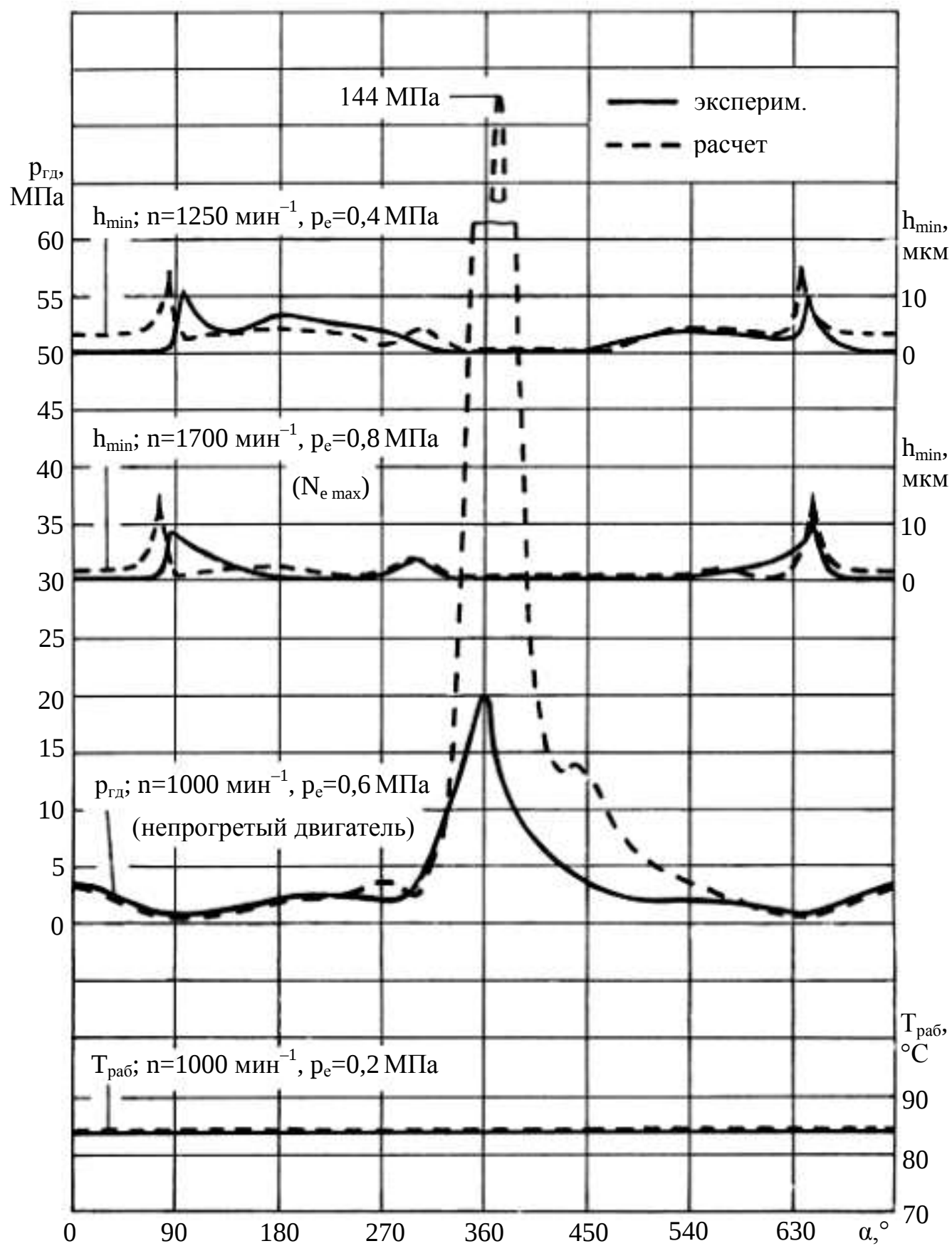
Рис. 4. Сравнение расчетных данных с экспериментальными
