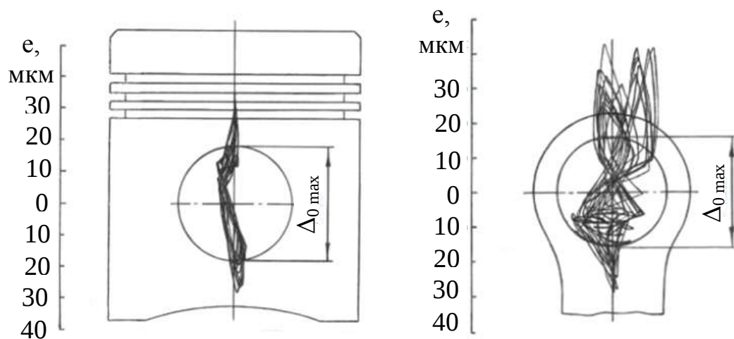
Рис. 2. Поля траекторий центра пальца в бобышке поршня и головке шатуна ( e – эксцентриситет)
