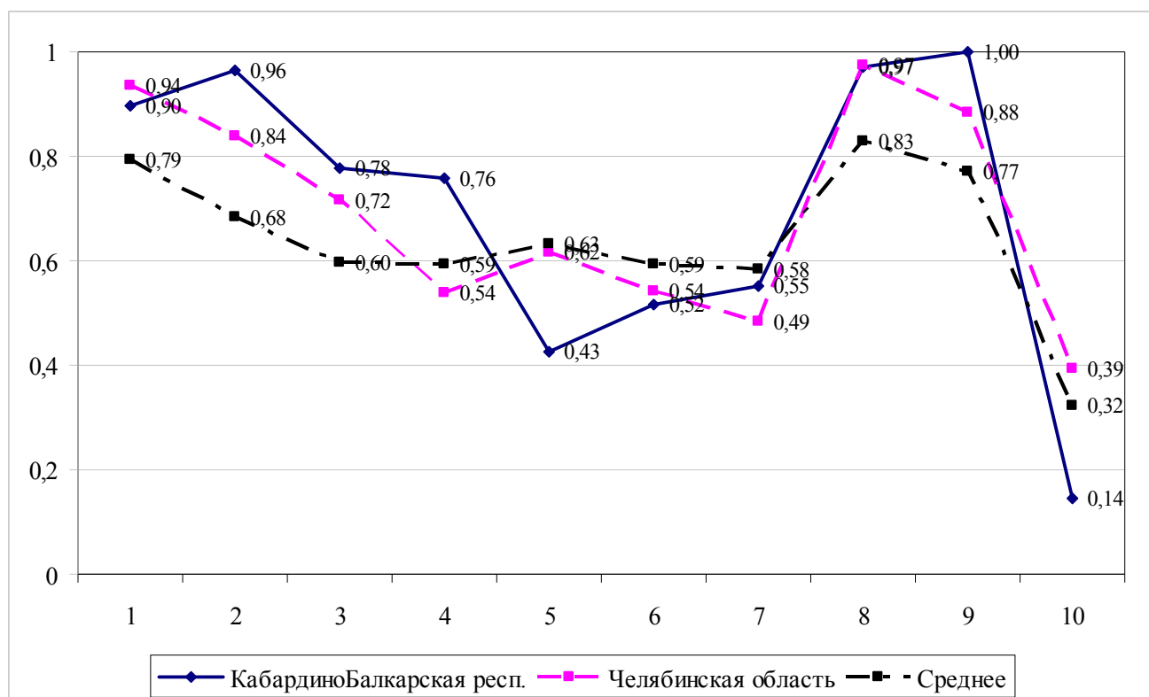
Рисунок 2 – Кривая эффективности (средние нормированные значения признаков)
