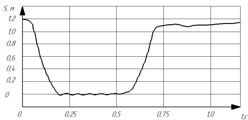
Рис. 8. Временная зависимость S(t) колебаний отдельного трака гусеницы по контуру гусеничного обвода
