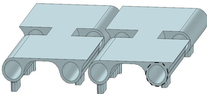
Рис 12. Разработанный вариант трака со смещением плит относительно друг друга и без обрезинивания беговой дорожки (гребни не показаны)
