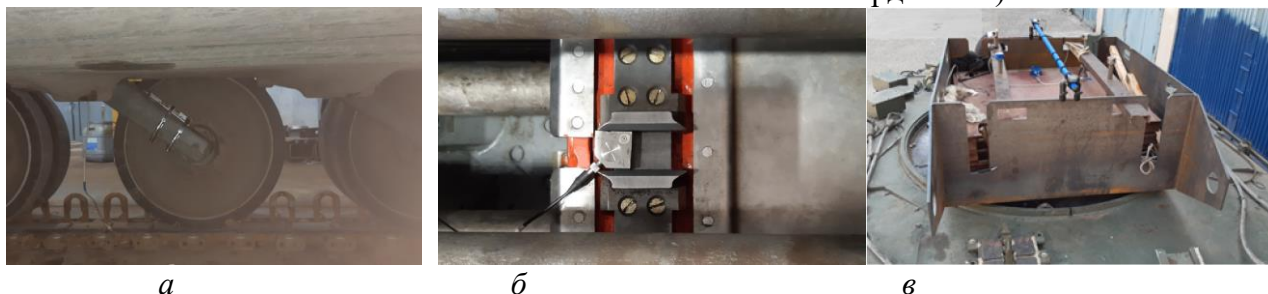
Рис. 7. Установка датчиков первичных преобразователей при экспериментальном исследовании динамической и виброакустической нагруженности: а – датчик ускорения на балансир опорного катка; б – датчик ускорения на раму держателя; в – спутниковые антенны, высокочастотный и низкочастотный датчики ускорения и датчик угловых скоростей на корпусе весового макета
