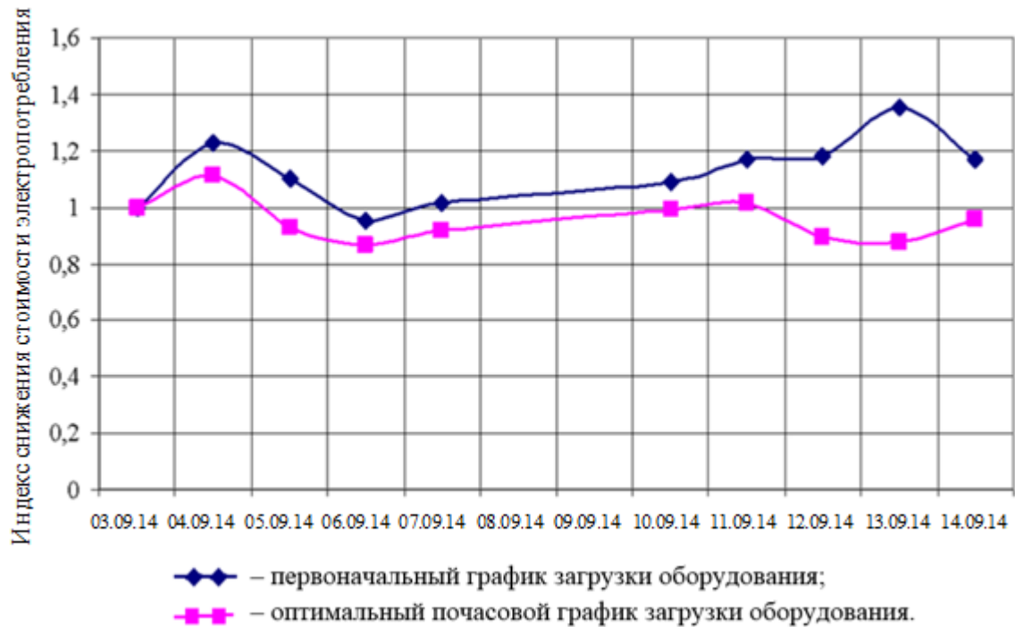
Рис. 4.15. Сравнение динамики изменения I_{сн} во времени для первого базового графика и для первого базового графика со смещением
