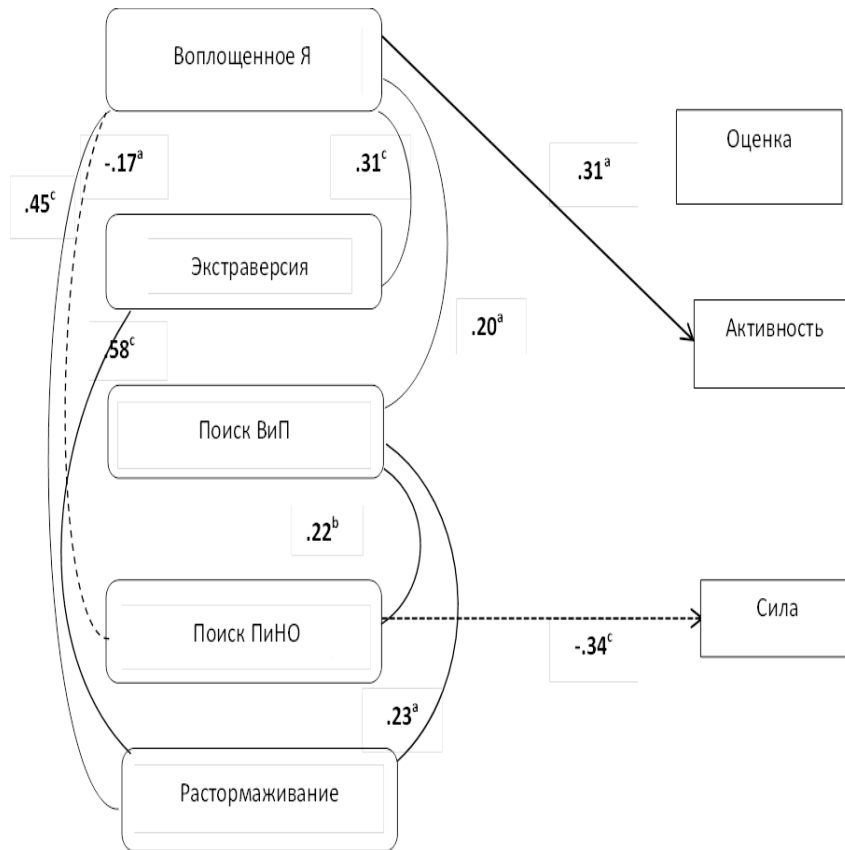
Рис. 1. Диаграмма путей структурной модели SM_1
