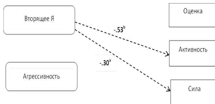
Рис. 4. Диаграмма путей структурной модели SM_4
