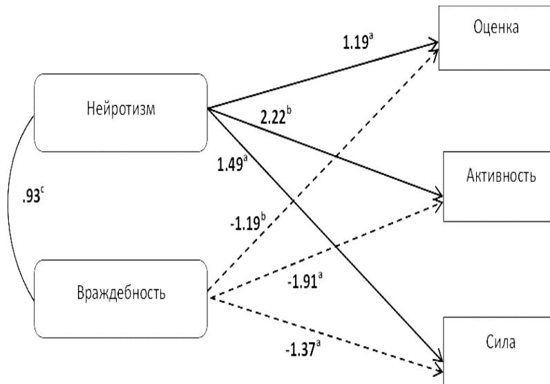
Рис. 2. Диаграмма путей структурной модели SM_2
