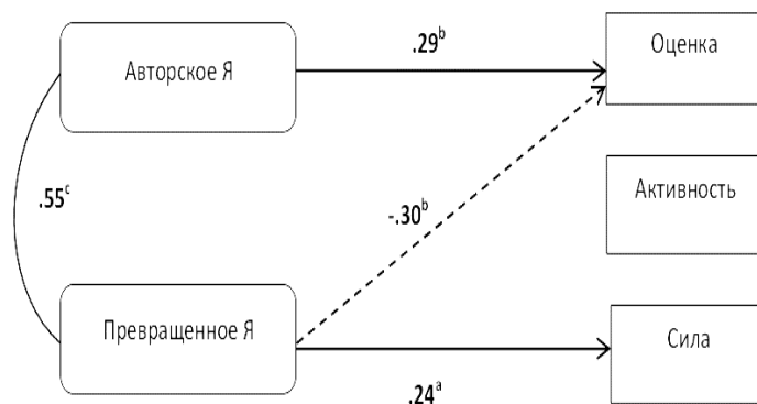
Рис. 3. Диаграмма путей структурной модели SM_3
